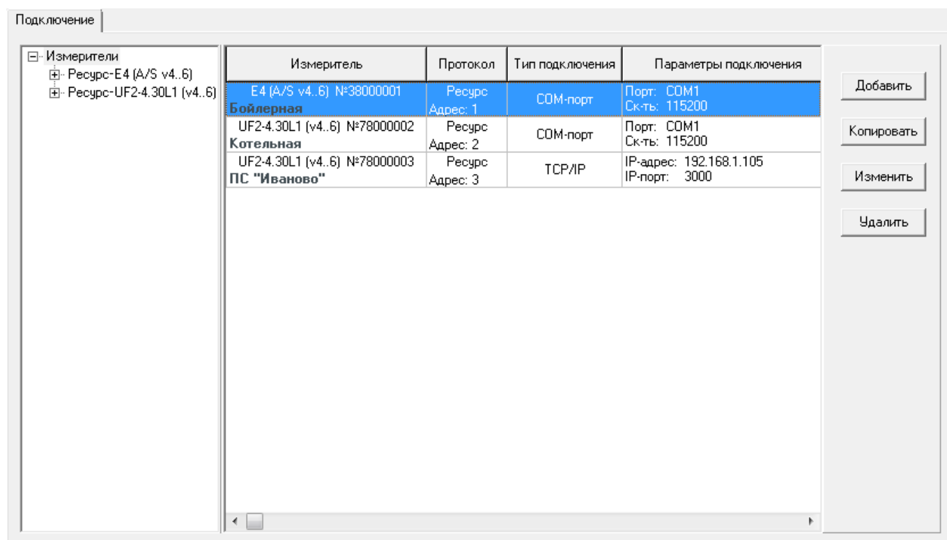
Рисунок 4.6 – Вкладка "Подключение". Все измерители
