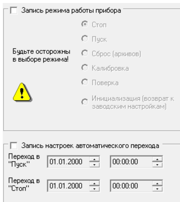
Рисунок 4.18 – Закладка "Режим работы"
